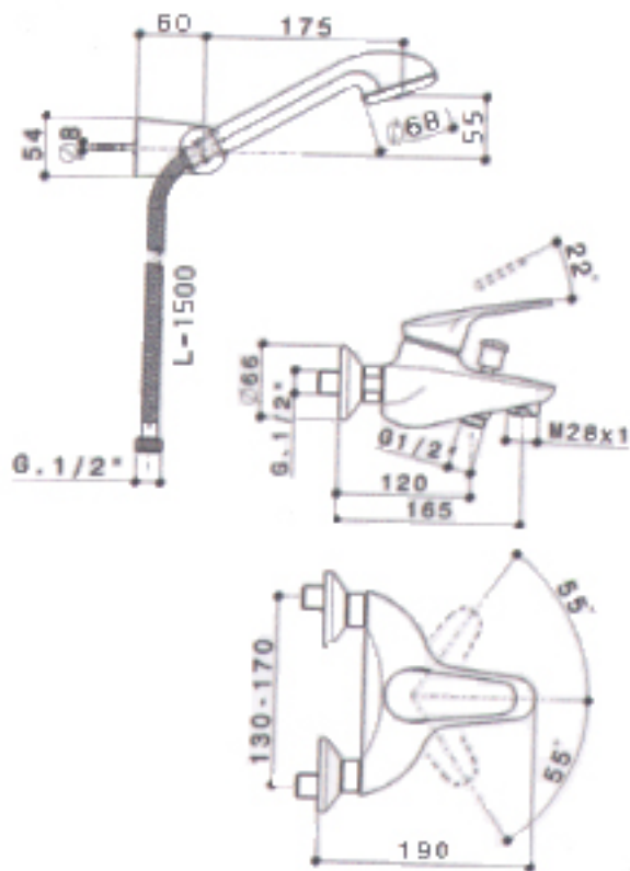
Mitigeur Bain Douche série Amilcar
